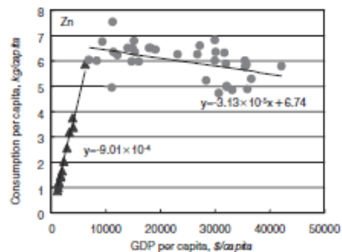
Fig. 4-9 Zinc
