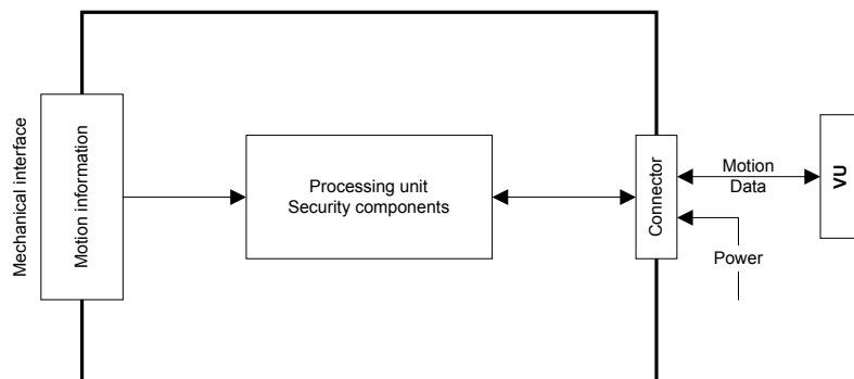
Figuur 1 Standaardbewegingsopnemer
