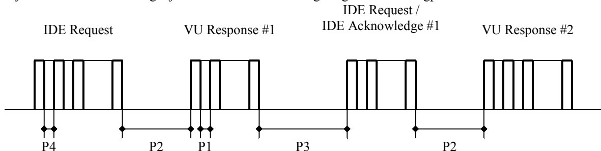
Figuur 1 - Berichtenstroom, timing
