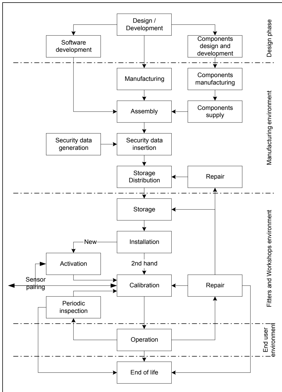
Figuur 3 Typische levenscyclus van de VU
