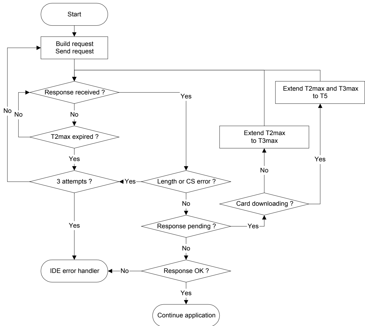
Figuur 3 - IDE behandeling van fouten
