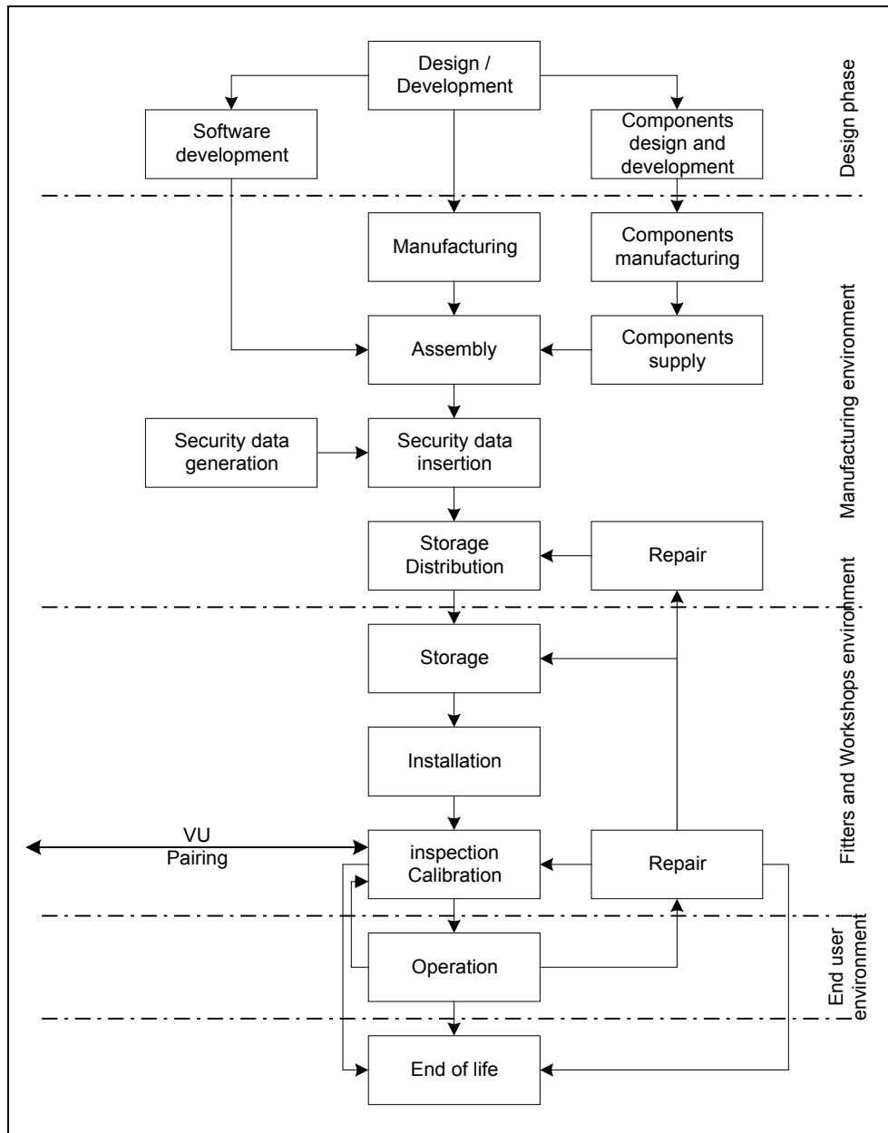
Figuur 2 Typische levenscyclus van de bewegingsopnemer
