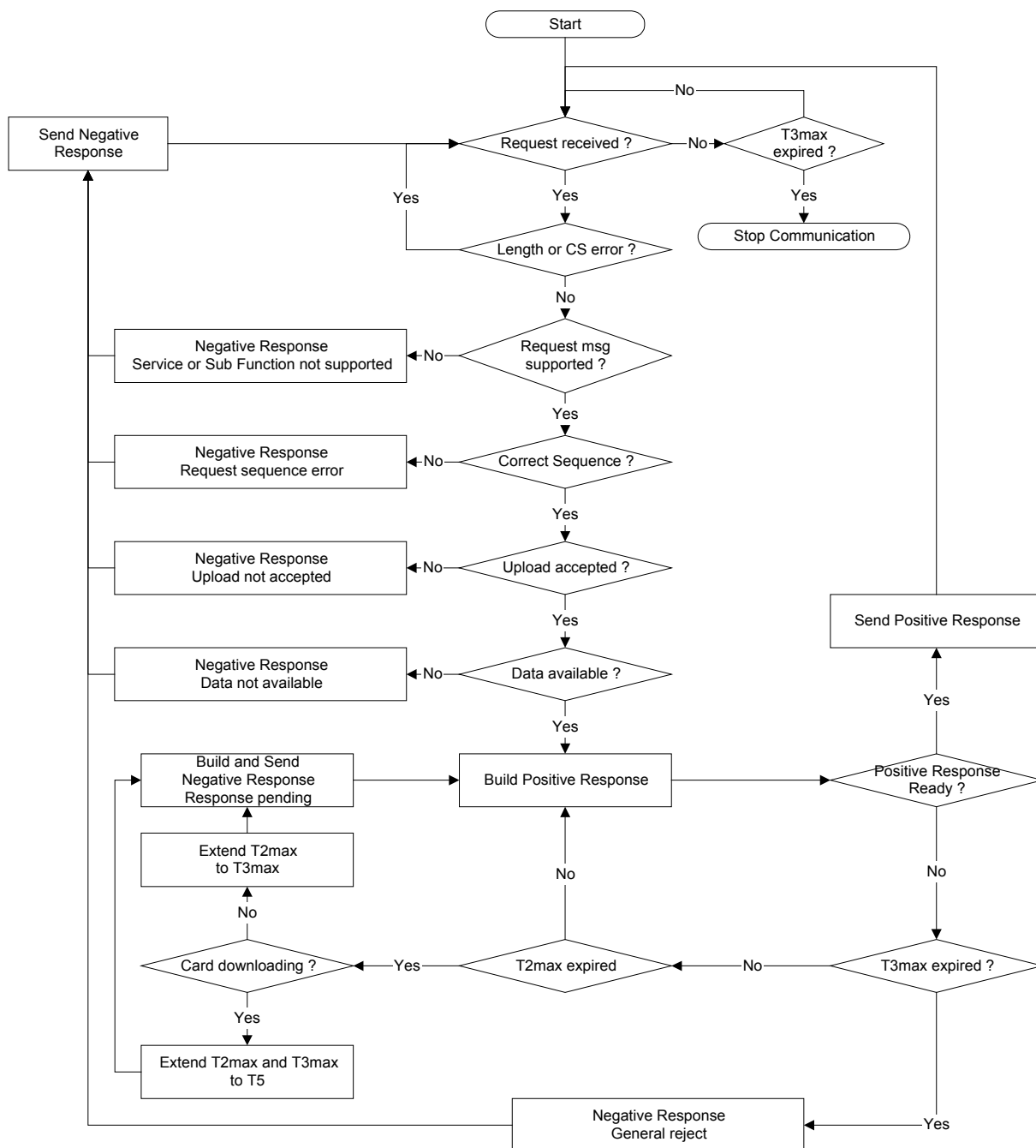
Figuur 2 - VU behandeling van fouten
