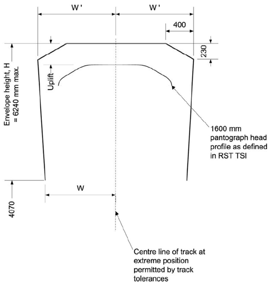
Figuur 7.5.2.7 — Omgrenzingsprofiel stroomafnemers
