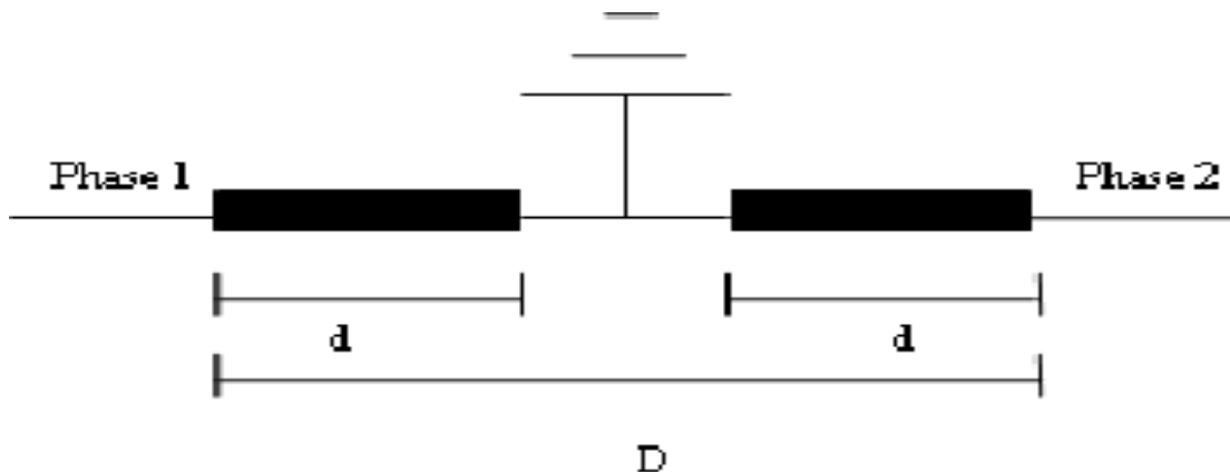
Figuur F.1: Scheidingssectie met neutrale sectie-isolatoren
