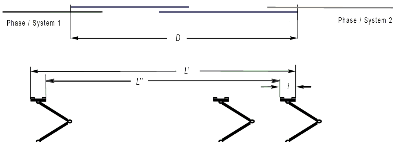
Figuur F.2– Gesplitste neutrale sectie
